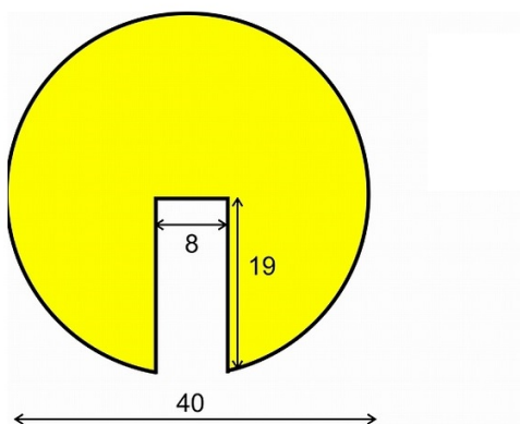
Protezione del bordo Tipo B
