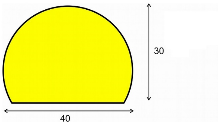
Protezione della superficie Tipo C
