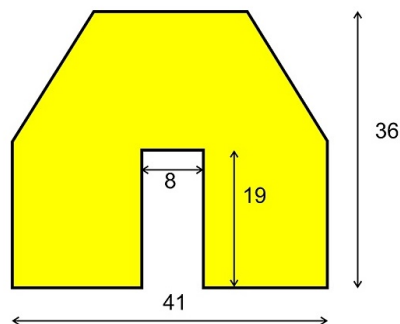
Protezione dei bordi tipo BB
